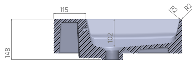
Sektion A-A
